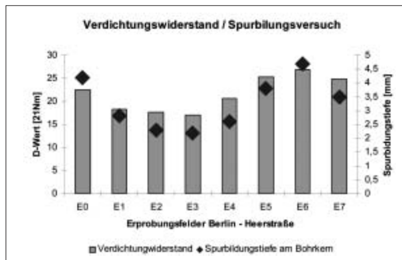
Abb. 3: Verdichtungswiderstand/Verformungsverhalten
