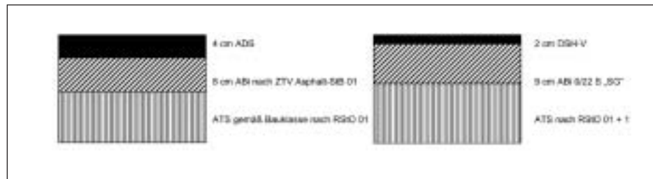
Abb. 4: Vergleich des alternativen Schichtenaufbaus mit einem konventionellen Aufbau nach RStO 01
