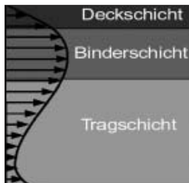
Abb. 1: Aufbau nach RStO 01 Schubspannungen unter Verkehr
